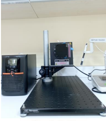
Güneş Simülatörü
